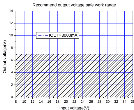
图 10.最大输出电压(IOUT=3000mA)
