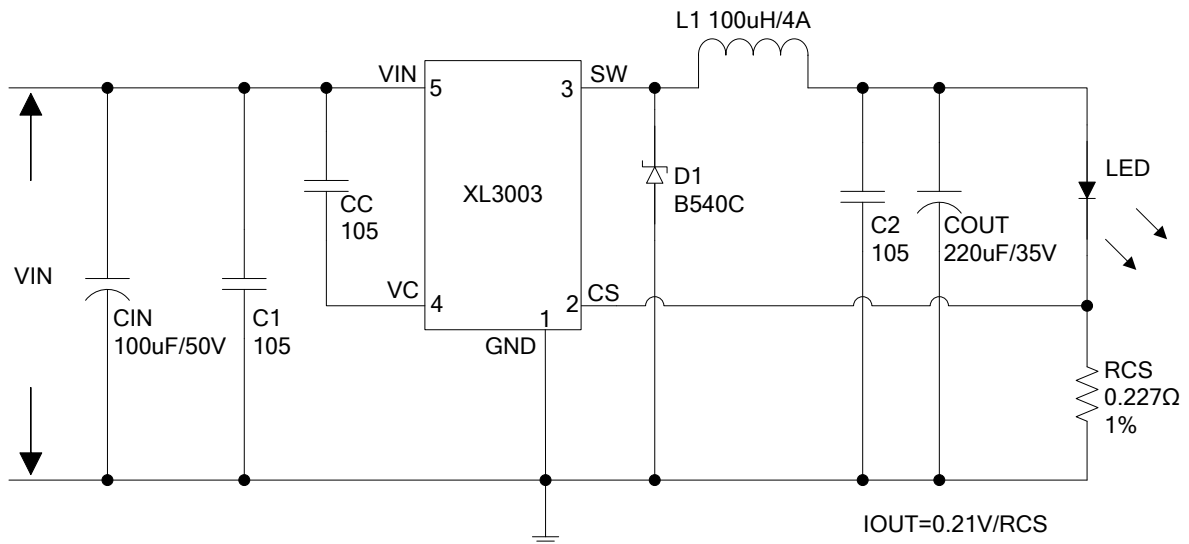
图 17. XL3003 系统参数测量电路 (VIN=8V~36V, IO UT =925mA)
