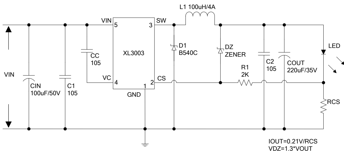
图20. XL3003系统参数测量电路 ( LED 开路保护 )
