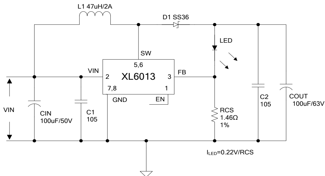
图 9.XL6013 系统参数测量电路 ( VIN=5V~40V,IO UT =150mA )
