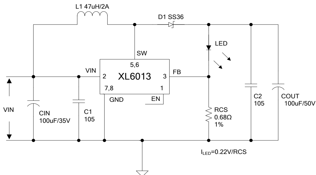
图 11. XL6013 系统参数测量电路 ( VIN=5V~30V,IOUT=320mA )
