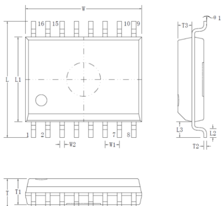
图 9. SOIC-16 封装
