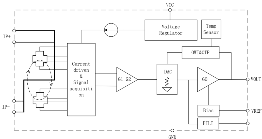
图 2. 功能框图
