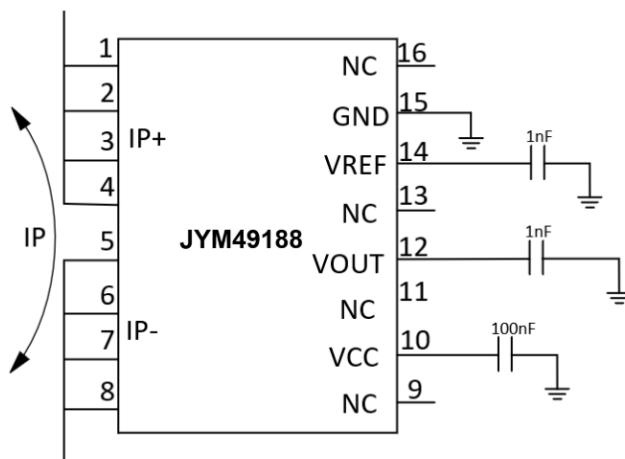
图 3. 应用电路
