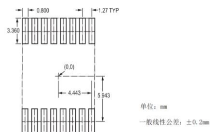
图 10. 推荐焊盘尺寸
