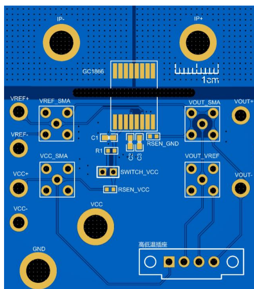
图 7.Demo 板正面
