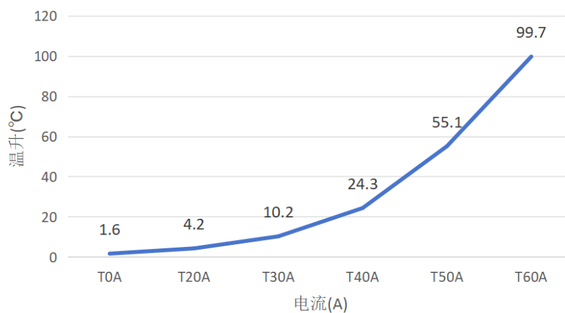
图 6.温升曲线图
