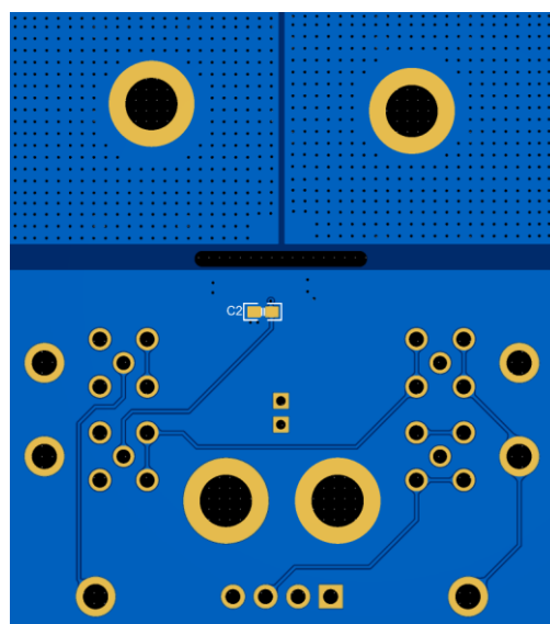
图 8.Demo 板反面
