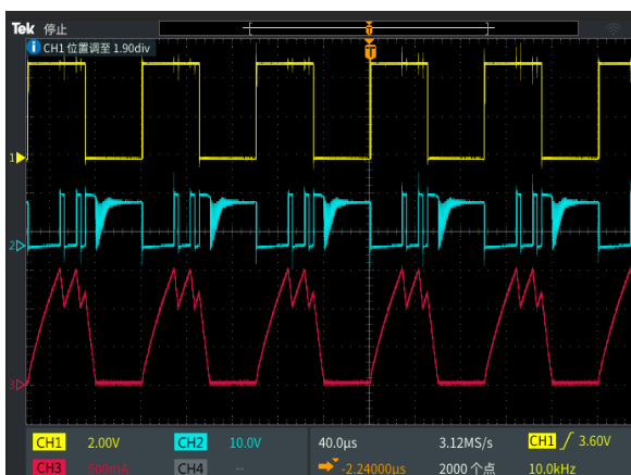
D=50% PWM 调光波形
