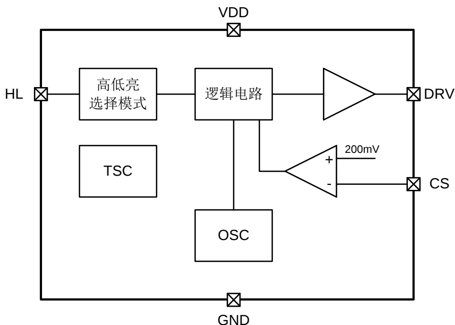
图 3. PT4125 内部模块简化图
