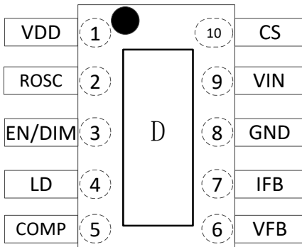
图 5.3 Hi6001 管脚图
