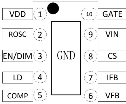
图 5.2Hi6000B 管脚图
