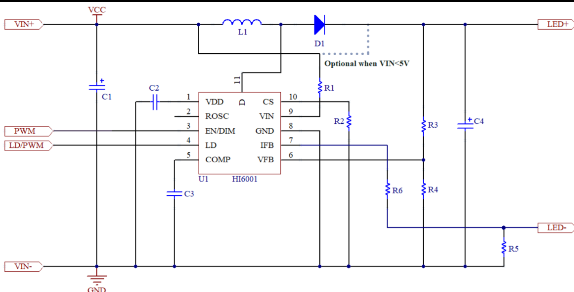
图 8.2 Hi6001 典型应用电路
