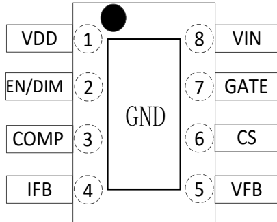
图 5.1 Hi6000A 管脚图
