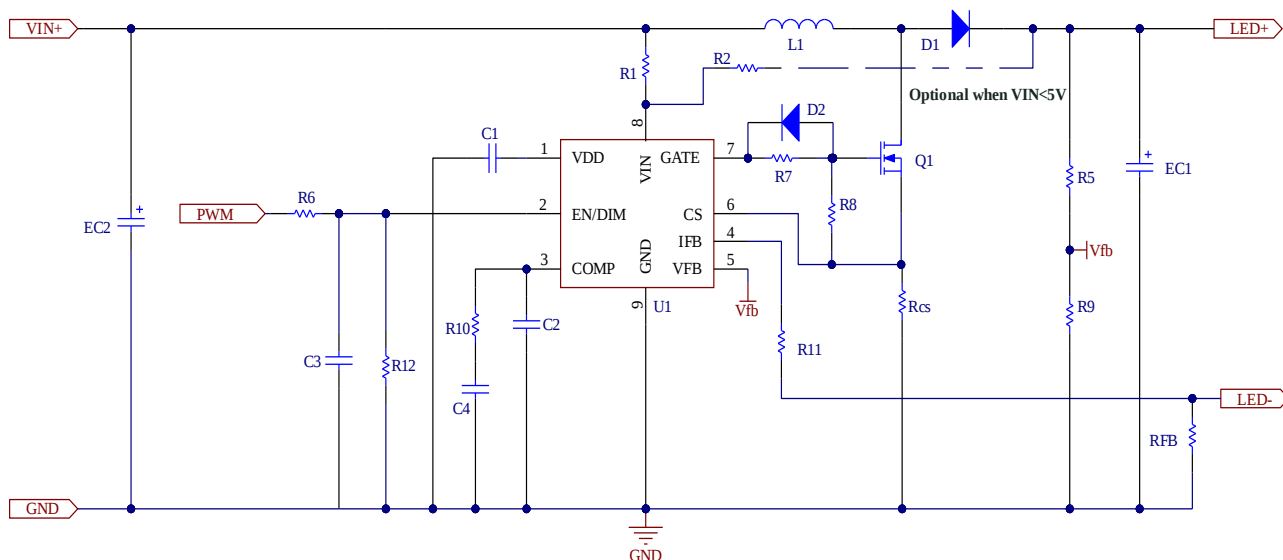
图 8.1 Hi6000A 典型应用电路
