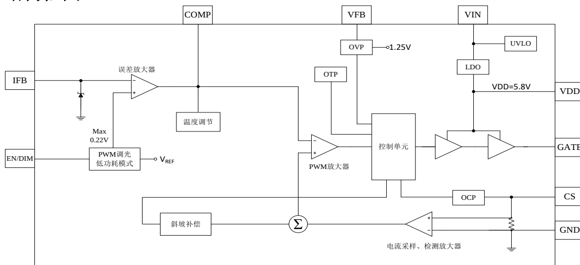
图 7.1 Hi6000A 芯片内部结构框图
