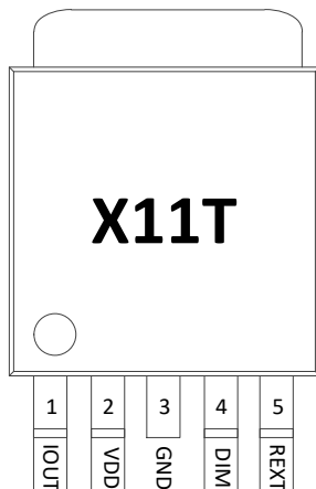
图 5.1 X11T 管脚图
