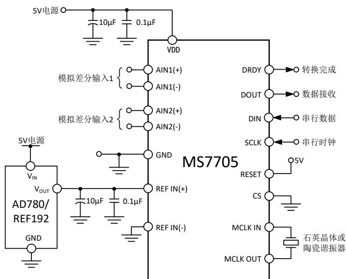
图 2. MS7705/MS7706 的基本连接电路图
