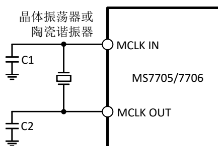
图 6. 晶体或陶瓷谐振器与 MS7705/MS7706 的连接
