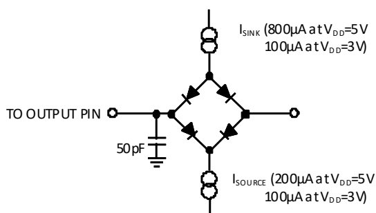
图 1. 负载电路（访问时间 and 总线释放时间）
