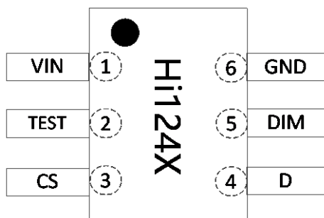
图 5 Hi124X 管脚图
