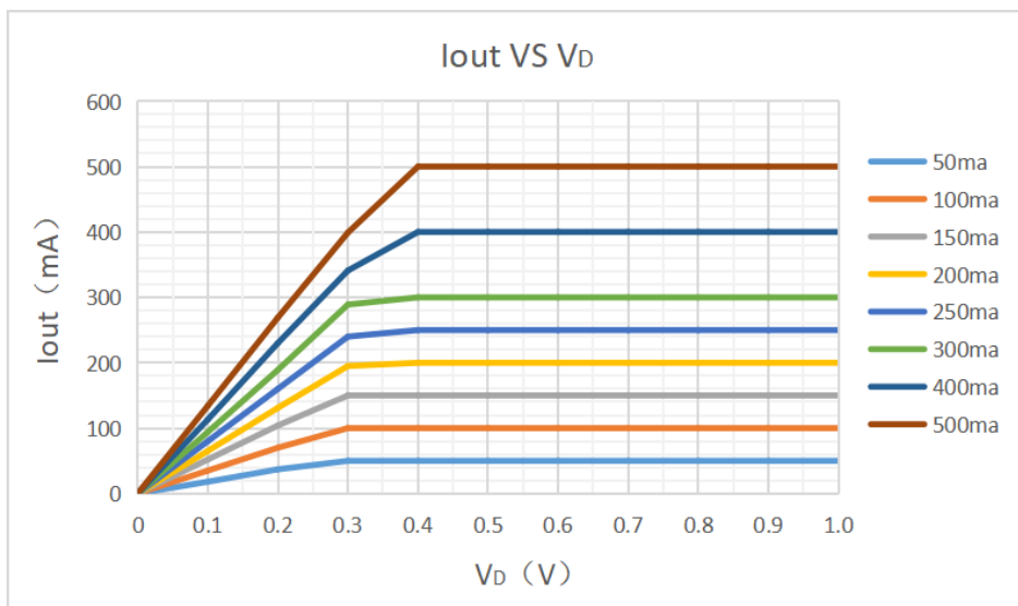
图 10.4 Hi15010 恒流拐点曲线
