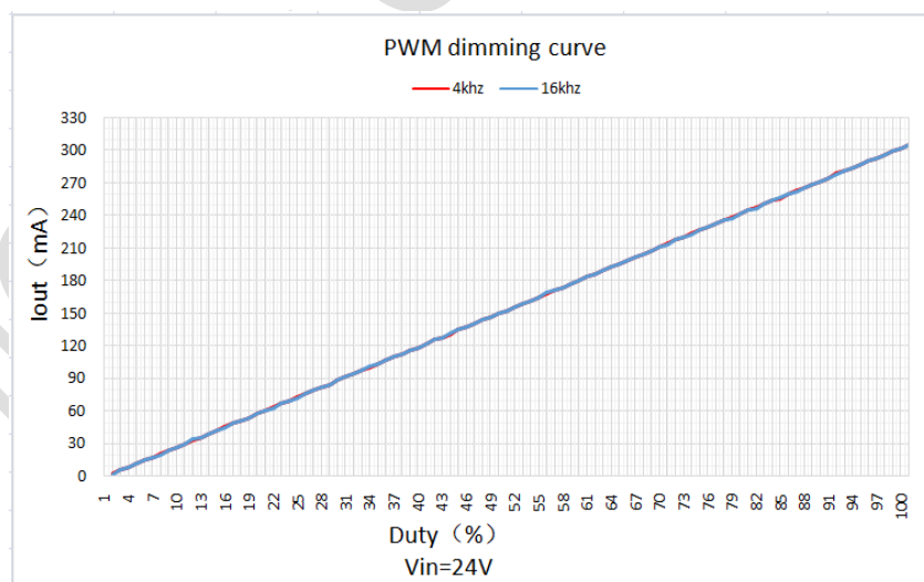
图 10.3 Hi15010 PWM 调光曲线
