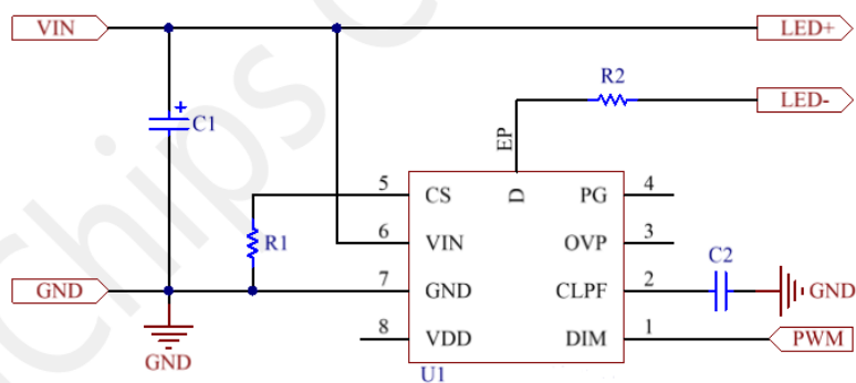
图 6.1 Hi150XE 应用电路
