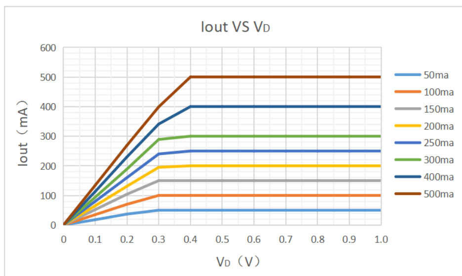
图 10.4 Hi150XE 恒流拐点曲线
