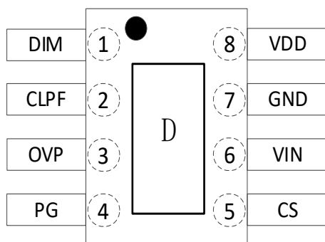
图 5 Hi150XE 管脚图
