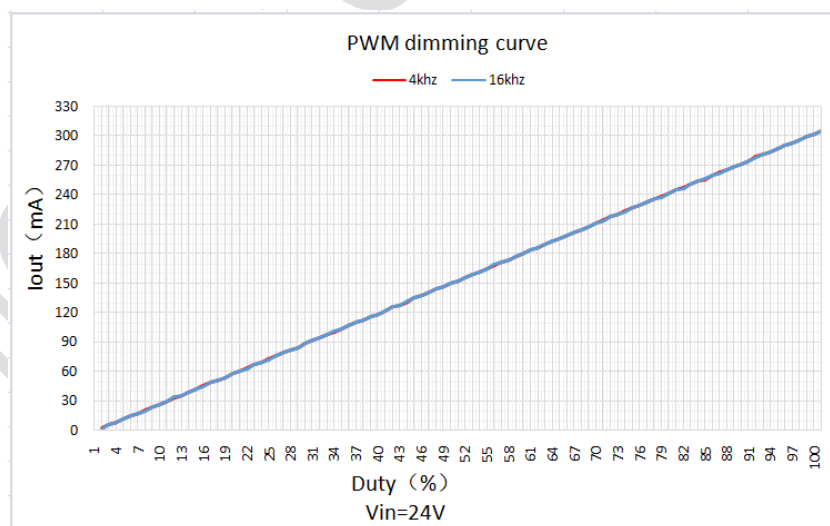
图 10.3 Hi150XE PWM 调光曲线
