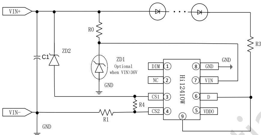
图 6.2 Hi12410W 过压保护电路
