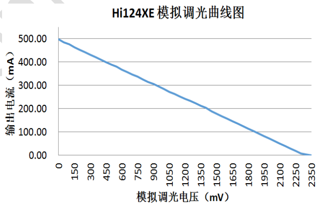
图 10.4.3 Hi124XE 模拟调光曲线
