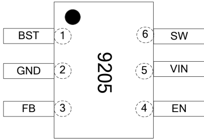
图 5.1 Hi9205 管脚图
