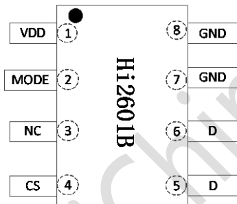
图 5.1 Hi2601B 引脚图
