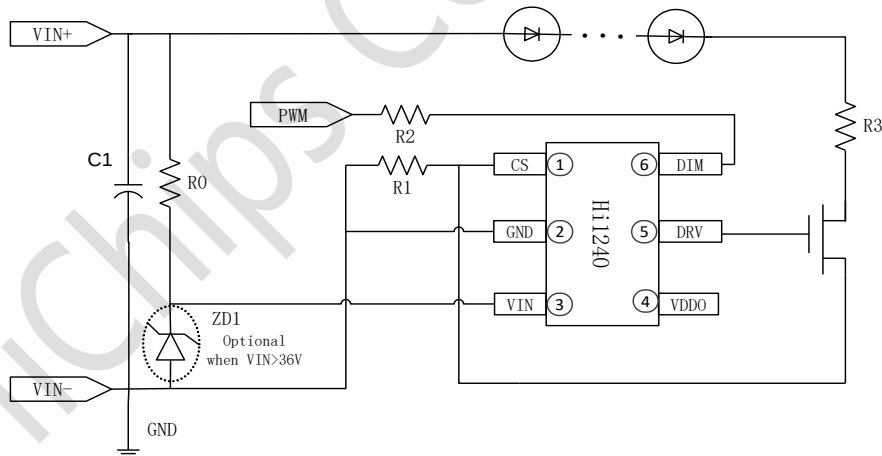
图 6 Hi1240 应用电路
