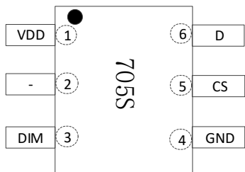
图 5.1 Hi7005S 管脚图
