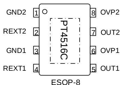
图 2. PT4516C 管脚定义图
