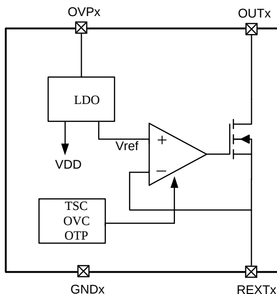
图 3. PT4516C 内部模块简化图
