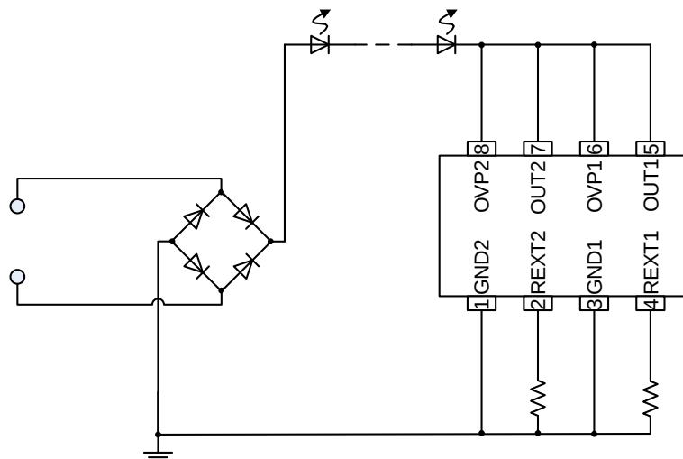
图 1. PT4516C 典型应用电路图
