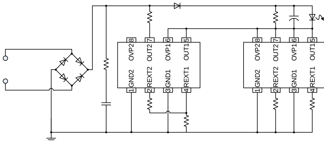
图 4. PT4516C TRIC 调光应用电路原理图
