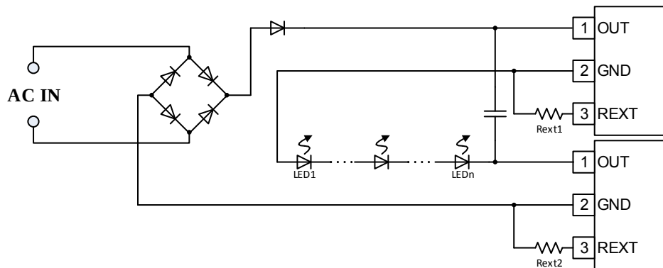
图 7. PT4515G 填谷电路应用电路原理图 2
