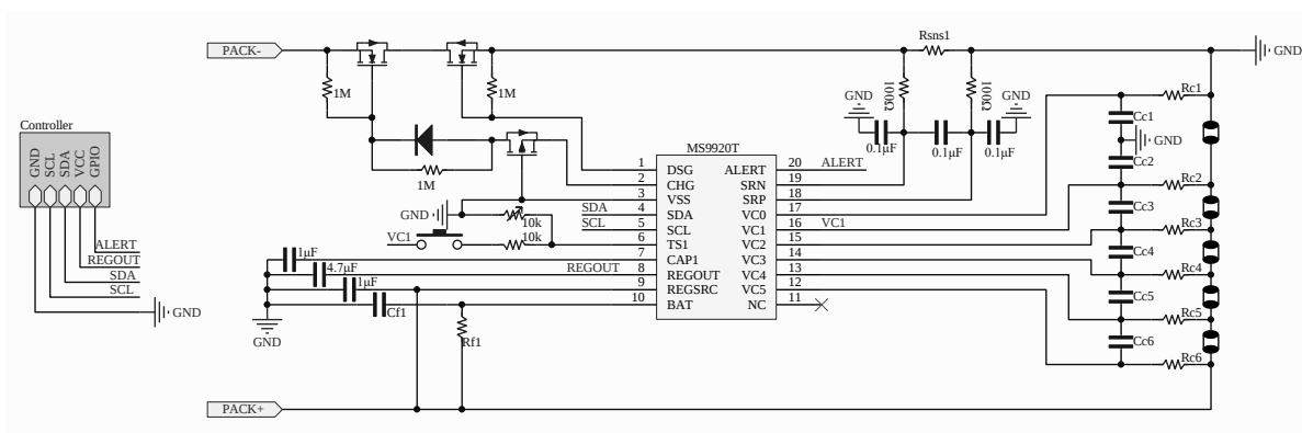
MS9920T 典型应用图
