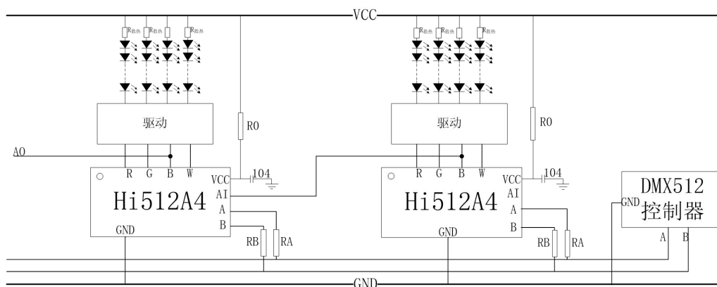
图 4.1 Hi512A4 应用示意图
