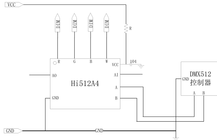
图 10.2.1 应用原理
