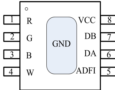
图 5.1 管脚图
