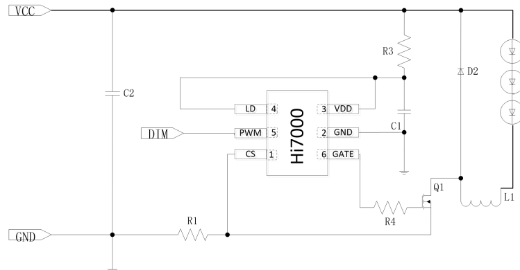
图 10.2.4 大功率 DCDC 典型应用
