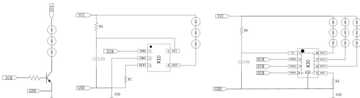
图 10.2.2 线性恒流应用
