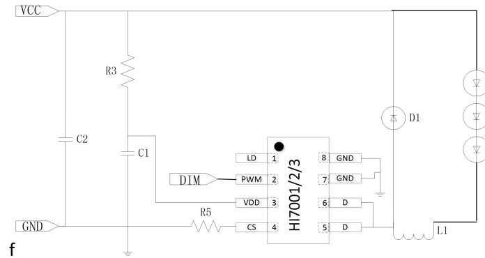
图 10.2.3 DCDC 典型应用
