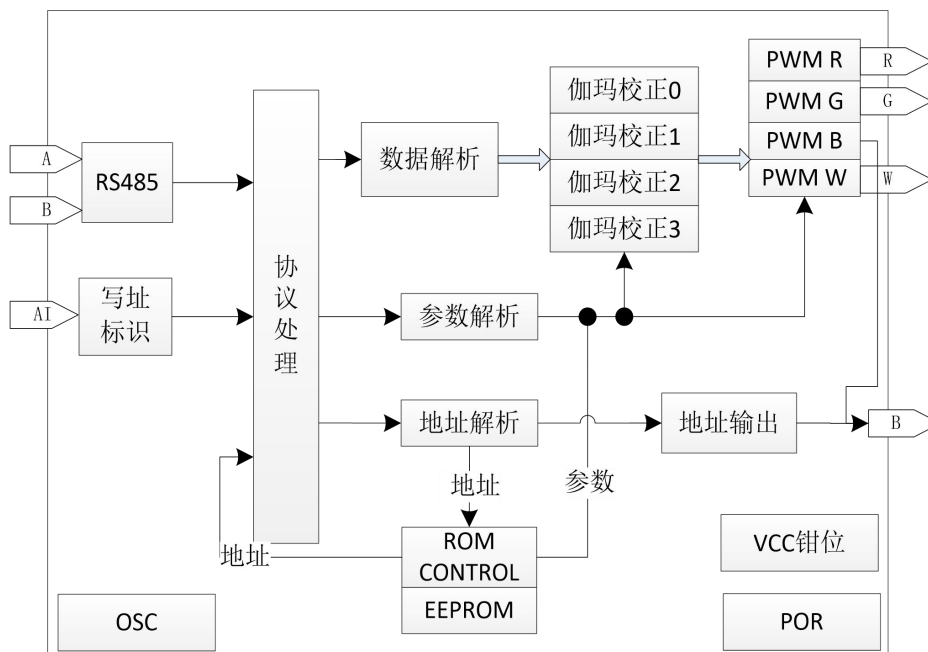
图 7.1 结构框图
